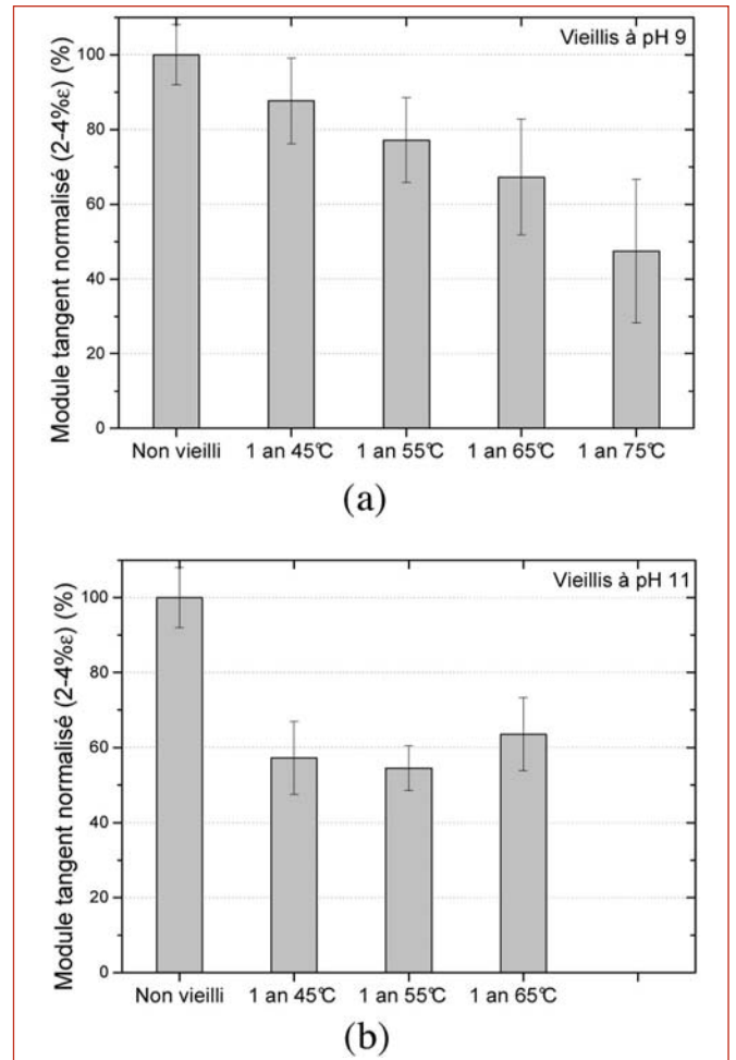
Figure 6 : Évolution du module tangent normalisé (2 et 4 % e) en fonction du temps de vieillissement de PET non vieillis et vieillis pendant 1 an à 45, 55, 65 et 75°C à pH 9 (a) et à pH 11 (b).
