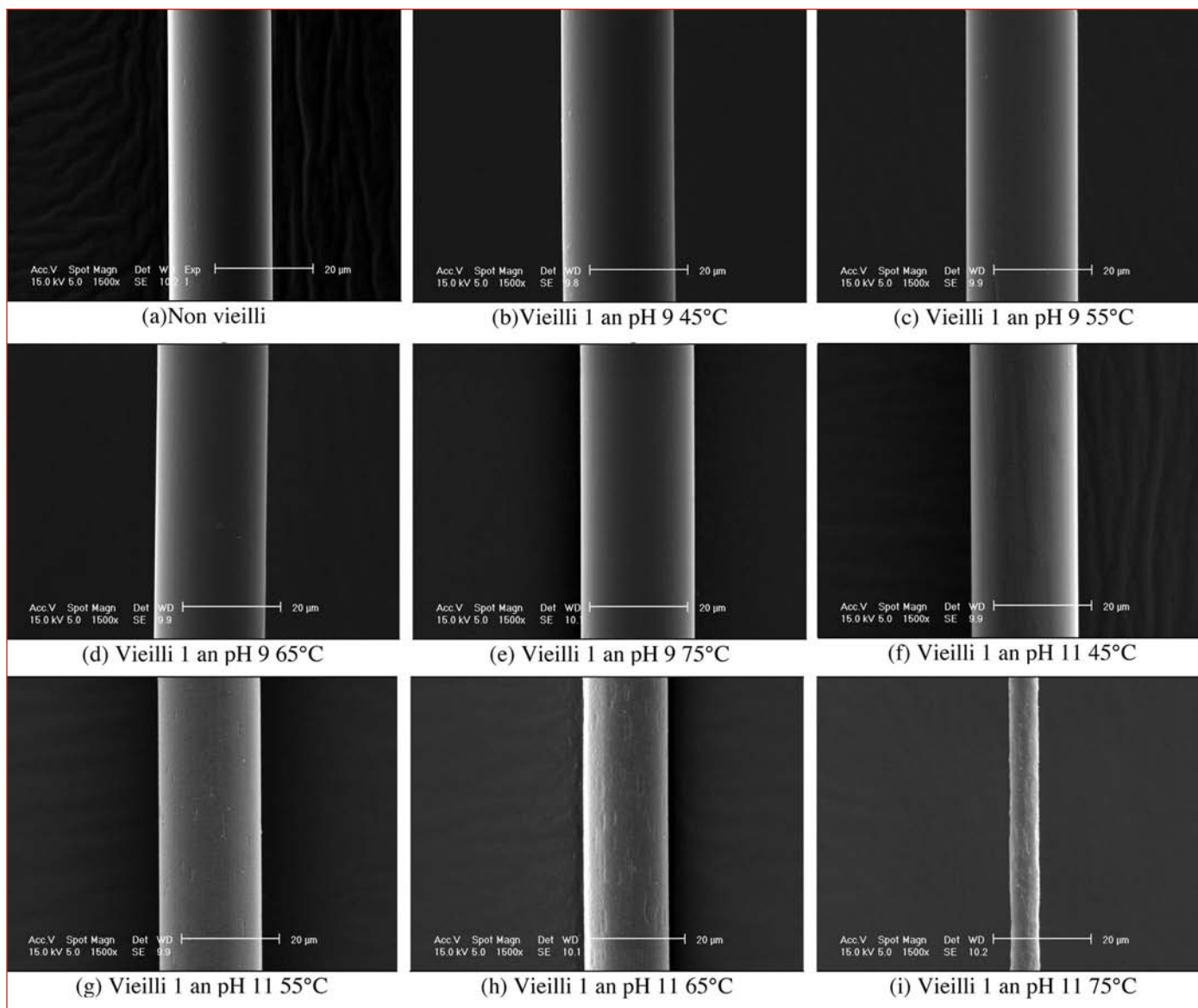
Figure 4 : Images de microscopie électronique à balayage (mode d'analyse en électrons secondaires) fibres de PET (a) non vieillis, vieillis 1 an à pH 9 (b) 45°C, (c) 55°C, (d) 65°C, (e) 75°C et vieillis 1 an à pH 11 (f) 45°C, (g) 55°C, (h) 65°C, (i) 75°C.
